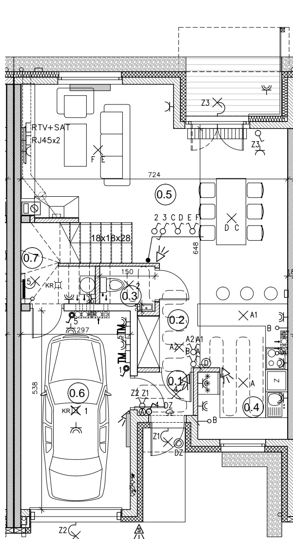
RZUT PARTERU
