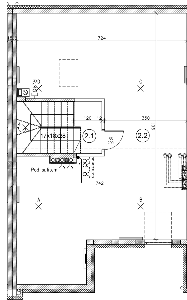
RZUT PODDASZA
