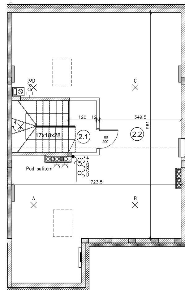
RZUT PODDASZA
