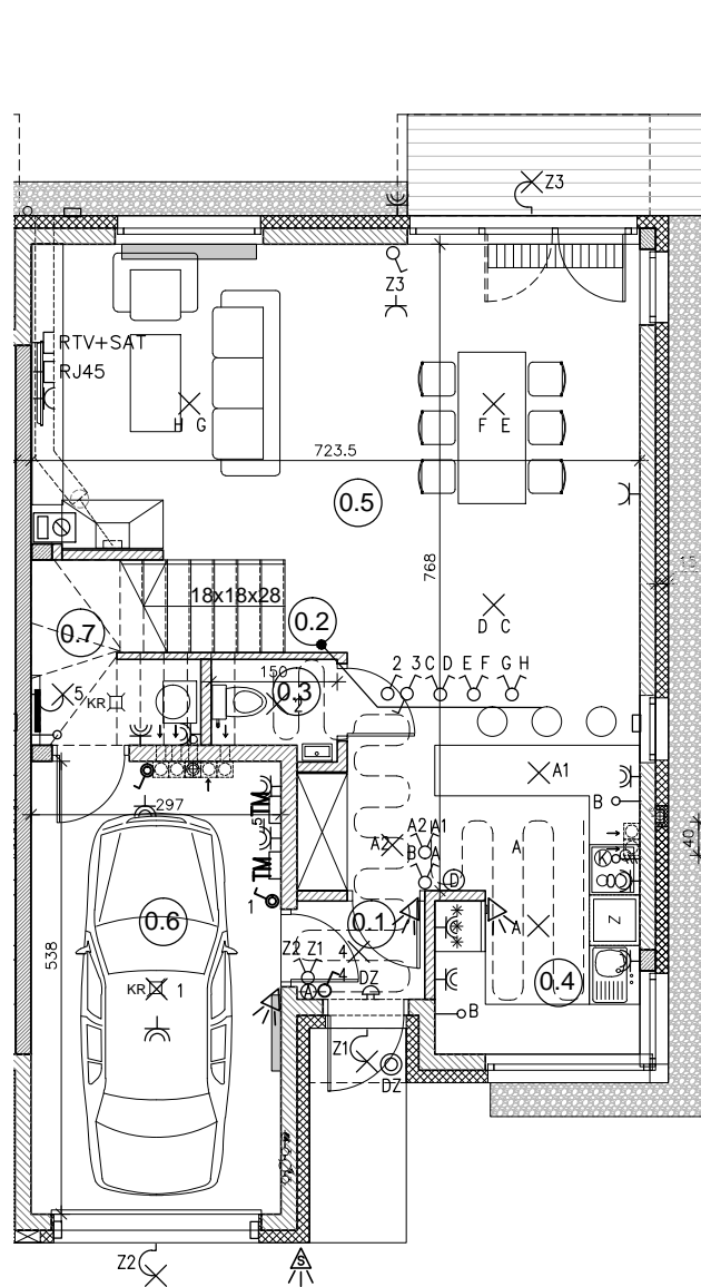
RZUT PARTERU
