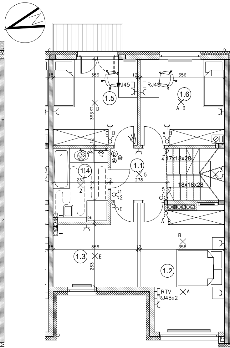
RZUT PIĘTRA
