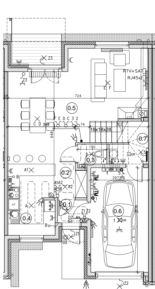
RZUT PARTERU
