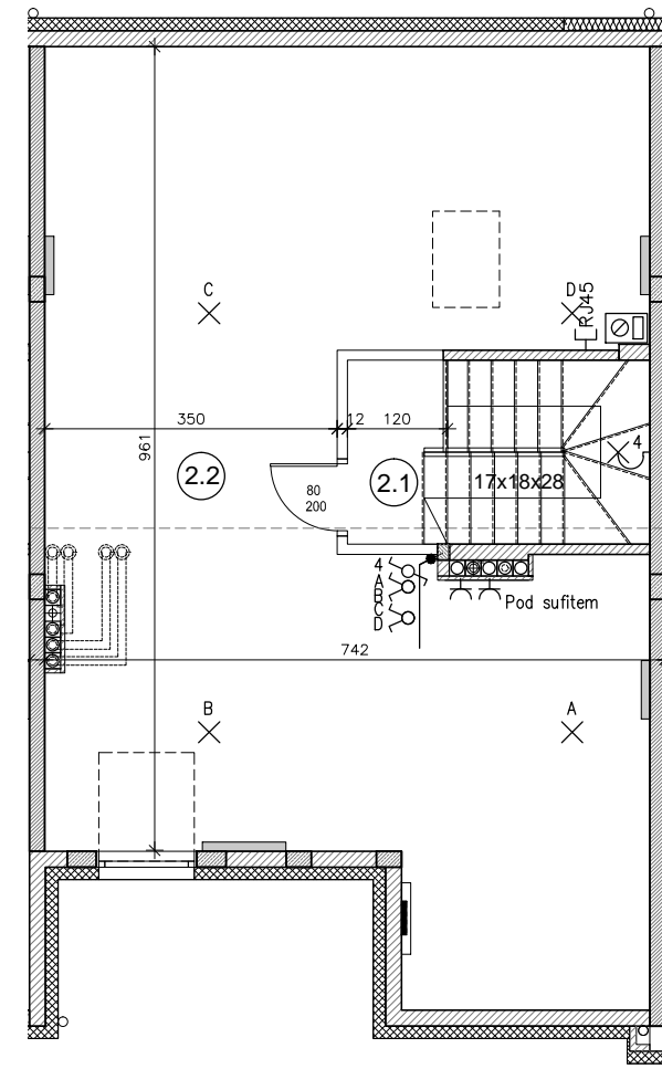
RZUT PODDASZA
